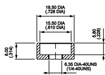
U825 For caps U630 & U3400
