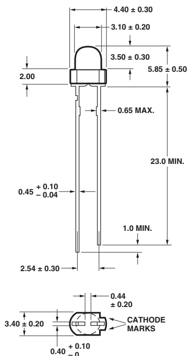
HLMP-NS30/NM31
