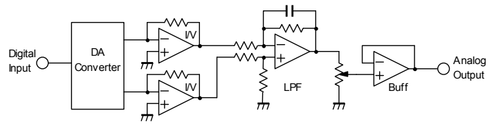
(Fig.2:DAC Output)
