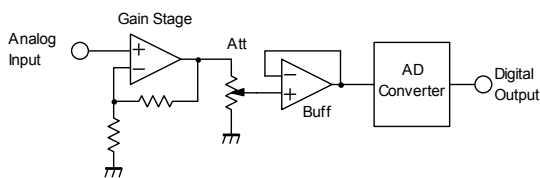
(Fig.1:ADC Input)
