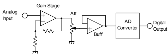
(Fig.1:ADC Input)
