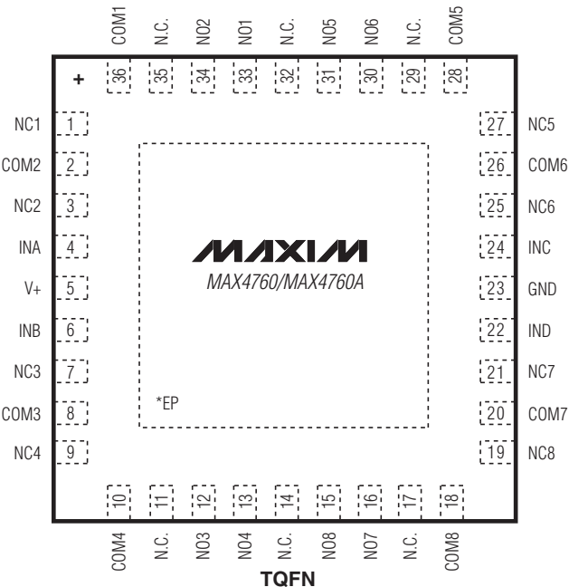
TQFN
