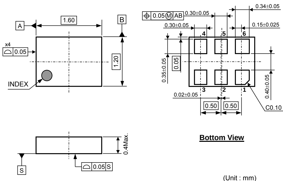
DFN(PLP)1216-6F Package Dimensions
