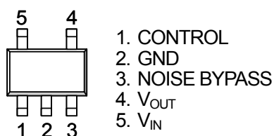
NJM2877F
