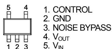
NJM2877F3
