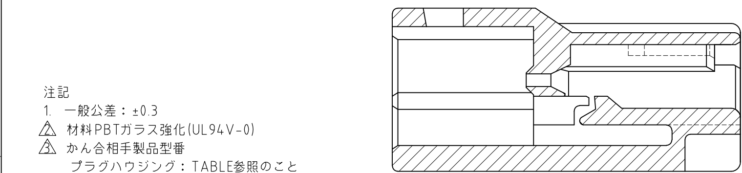
断面 A-A SECT A-A
