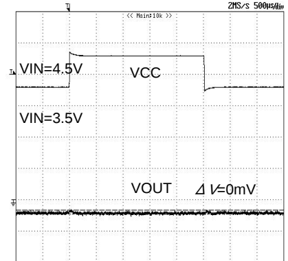
Fig.37 Transient_response (Ta=85°C)
