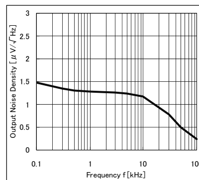
Fig.57 Noise - Freq.
