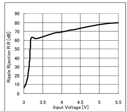
Fig.55 R.R. - VIN
