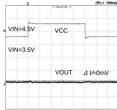
Fig.36 Transient_response (Ta=25°C)
