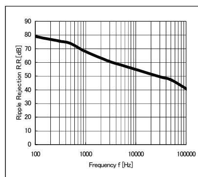
Fig.10 R.R. - Freq.
