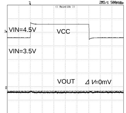
Fig.37 Transient_response (Ta=85°C)
