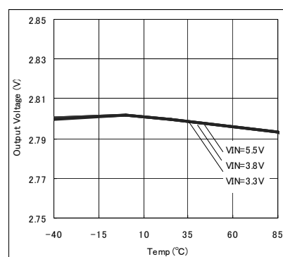
Fig.30 VOUT - Temp
