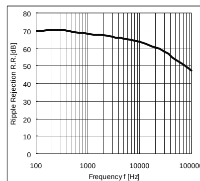
Fig.33 R.R. - Freq.
