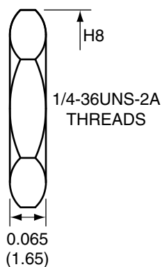
NUT
