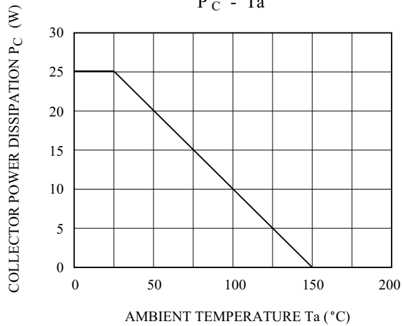
P_C - T_a
