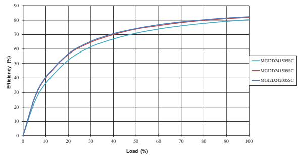
24V INPUT
