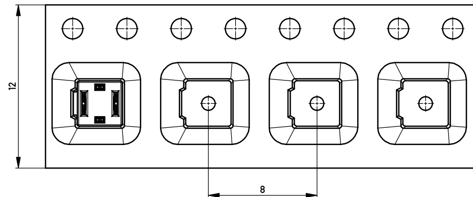
Abspulrichtung - Reel off Direction
