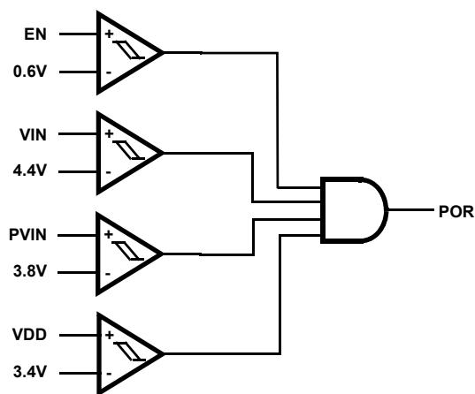
FIGURE 31. POR CIRCUIT
