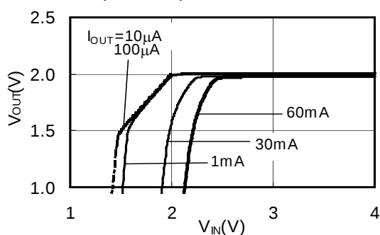
S-818A20A ( T_a=25^\circ\text{C} )
