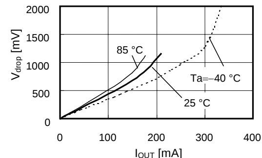
S-818A30A
