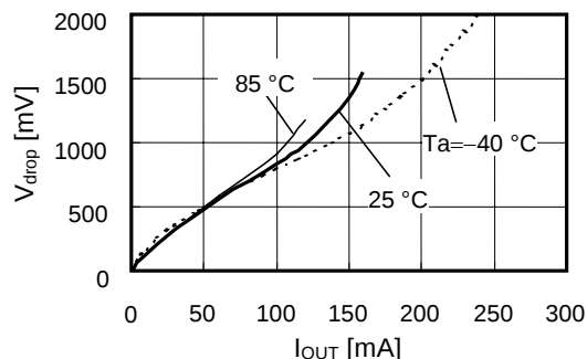
S-818A50A
