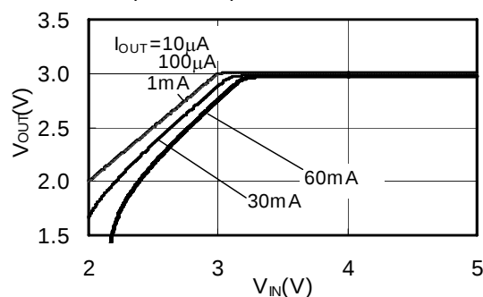
S-818A30A ( T_a=25^\circ\text{C} )
