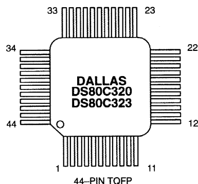
44-PIN TQFP
