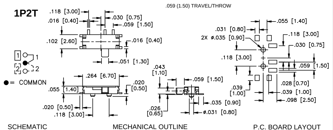
RIGHT ANGLE ACTUATOR
