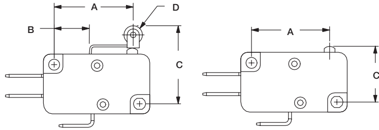
FIG. 1 Lever Roller
