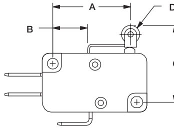
FIG. 1 Lever Roller
