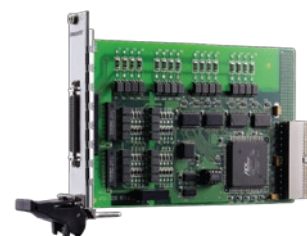
cPCI-7230
