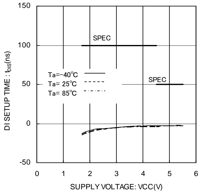
Figure 27. DI setup time t_{bis}
