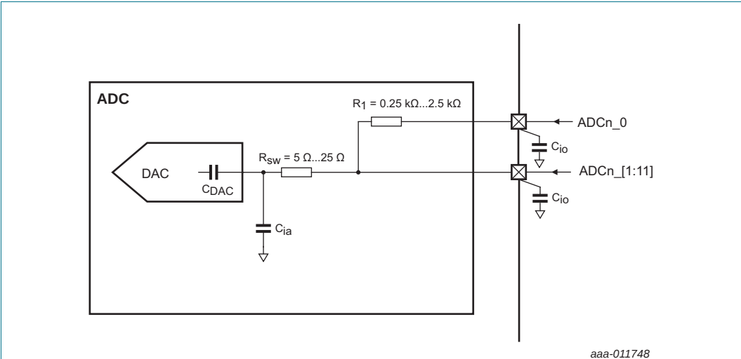
Fig 36. ADC input impedance
