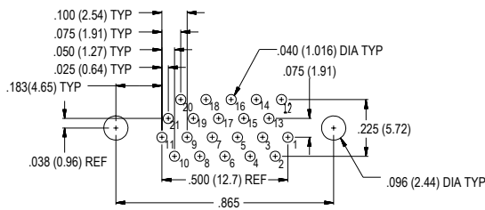
21 PIN MWDM-21PCBS
