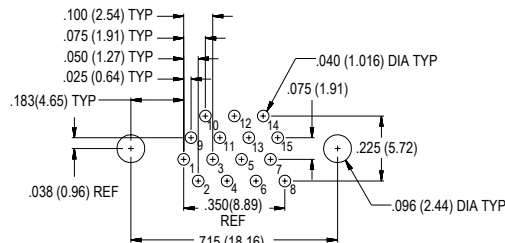
15 Socket MWDM-15SCBS
