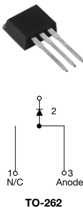
VS-30ETH06-1PbF
