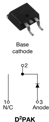
VS-30ETH06SPbF
