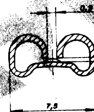
SECCÃO-A-A
