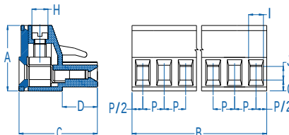
Dimensions
