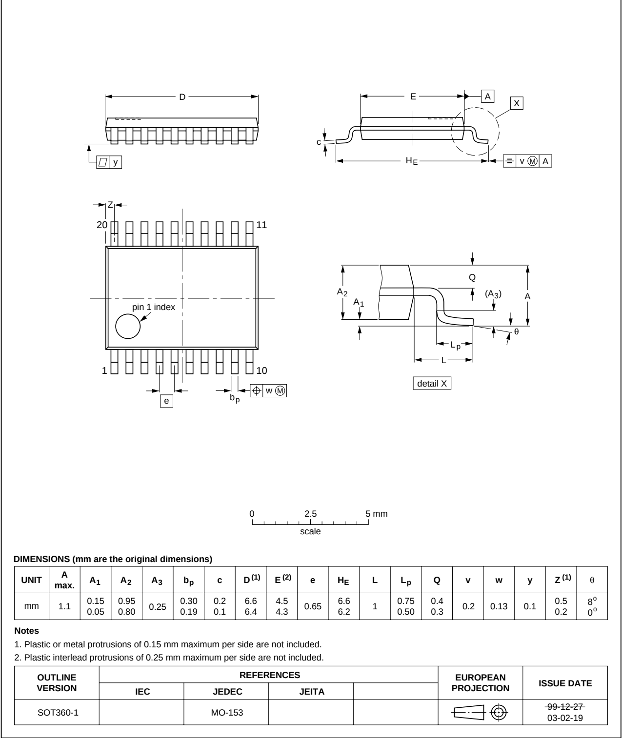
Fig 15. TSSOP20 (SOT360-1).
