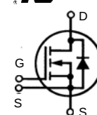
miniBLOC, SOT-227 B (IXFN)
