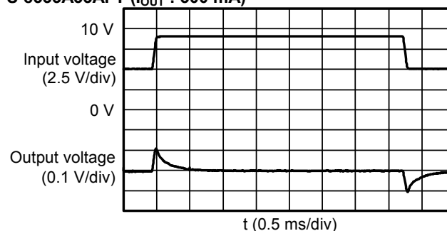
S-8533A50AFT ( I_{OUT} : 500 mA)
