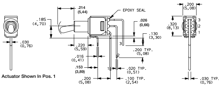
Actuator Shown In Pos. 1
