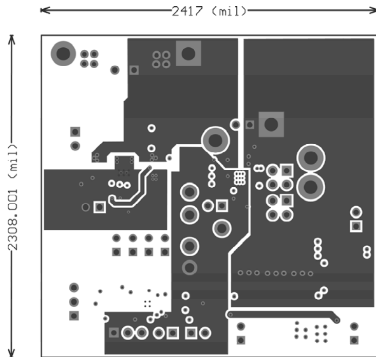
Copper Layer 3
