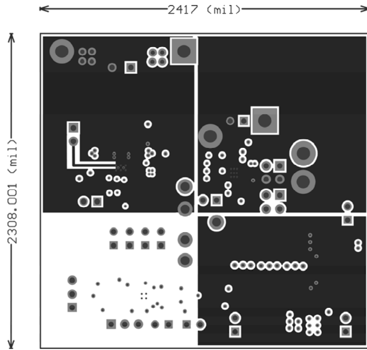
Copper Layer 2
