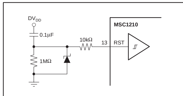
Figure 16. POR Circuit
