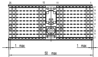
Lochbild fuer Leiterplatte (Bestueckungsseite) Board hole pattern (Component mounting side)
