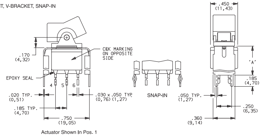
E201J1_BE2 DPDT
