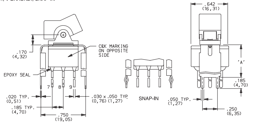
E301J1_BE2 3PDT
