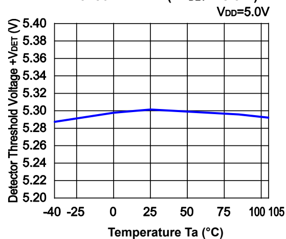
R3150NxxxE/F (+V DET = 5.3 V)
