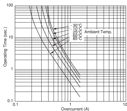
PTGL05AS6R8K3B51B0
