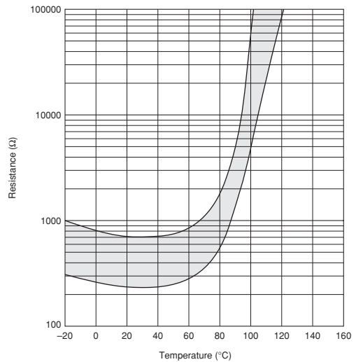
PRF18/21BD471Q Type
