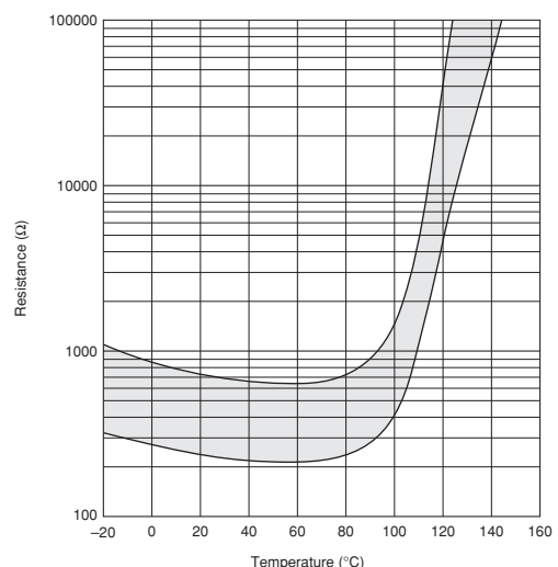
PRF18/21BB471Q Type
