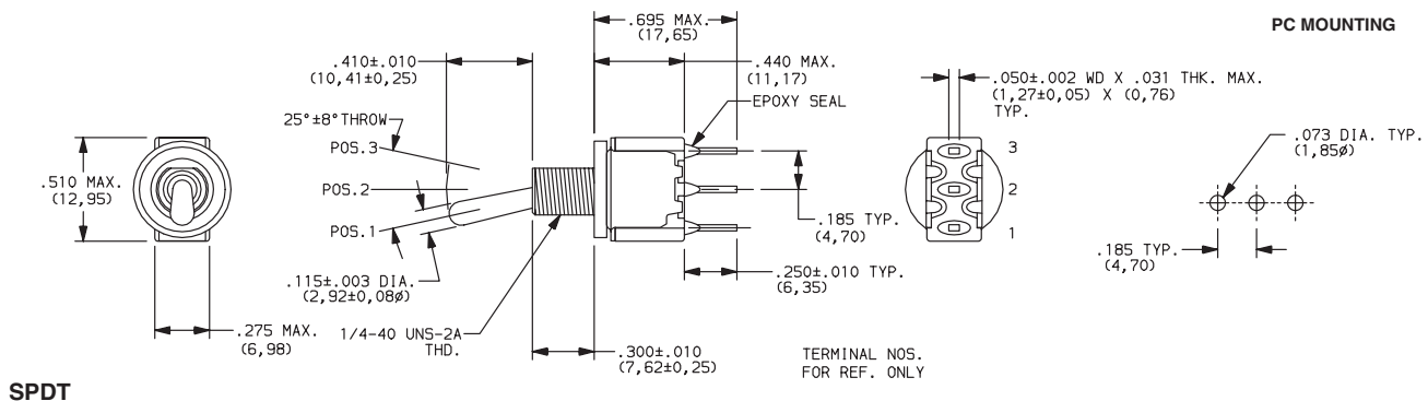
SPDT
