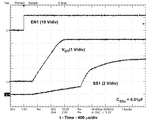
Figure 10. \text{VO1}=3.3\text{V} , SoftStart
