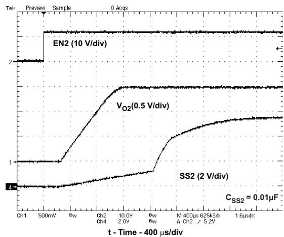
Figure 11. \text{VO2}=1.5\text{V} , SoftStart
