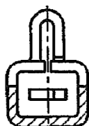
断面 "C" - "C" (SECT)
