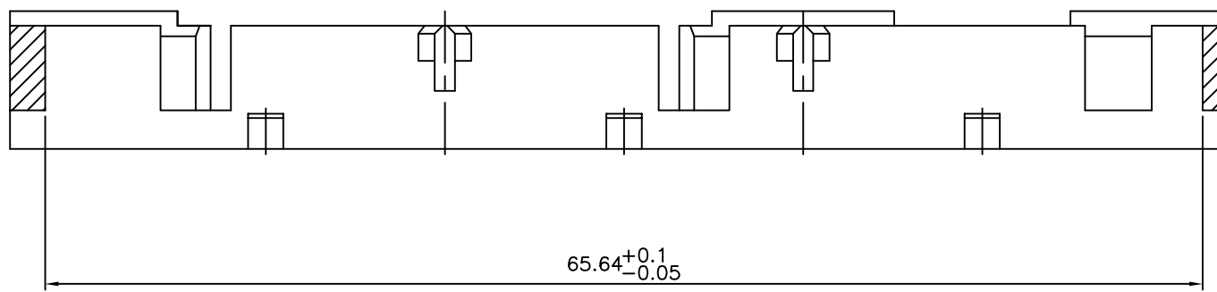
SECTION A-A
