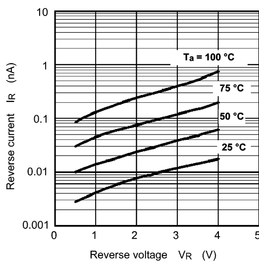
Fig. 9.2 I_R - V_R
