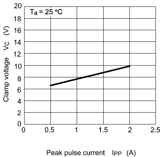
Fig. 6.3.1 V_C - I_{PP}
