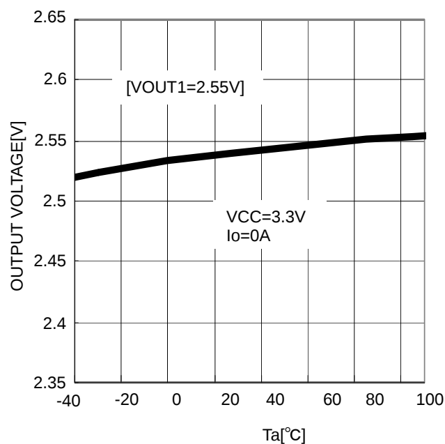
Figure.7 Ta-VOUT1
