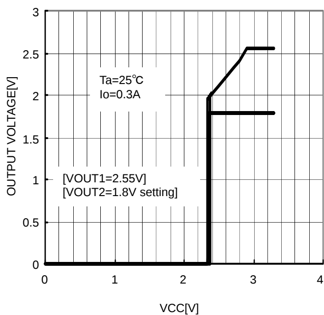
Figure.4 VCC-VOUT
