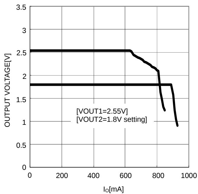
Figure.6 IOU-VOUT
