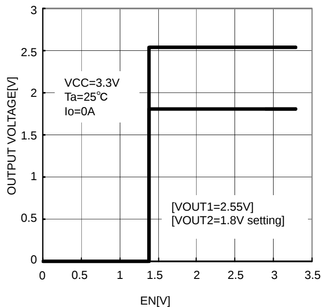
Figure.5 VEN-VOUT
