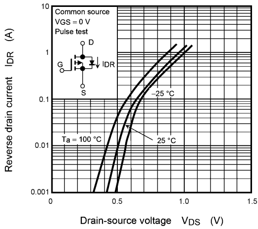
Fig. 7.9 I_{DR} - V_{DS}
