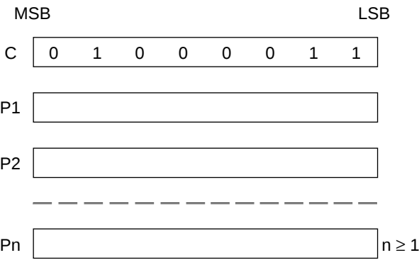
Figure 25. MREAD parameters
