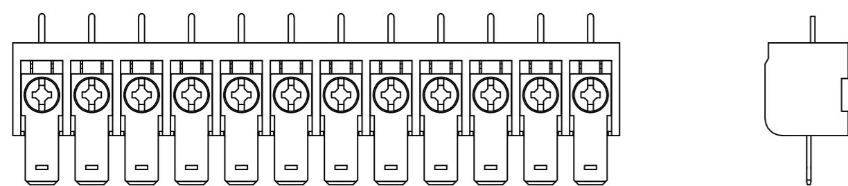
2-796988-9 OBSOLETE .250 TYP
